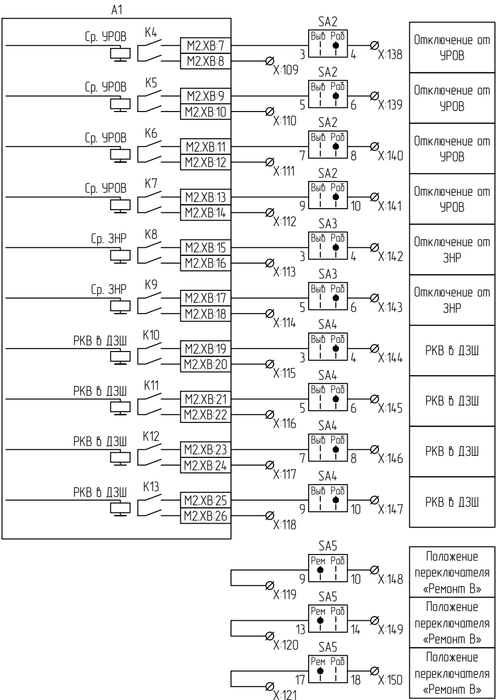
Выходные цепи
